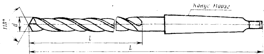
Вариант исполнения сверл с шейкой
