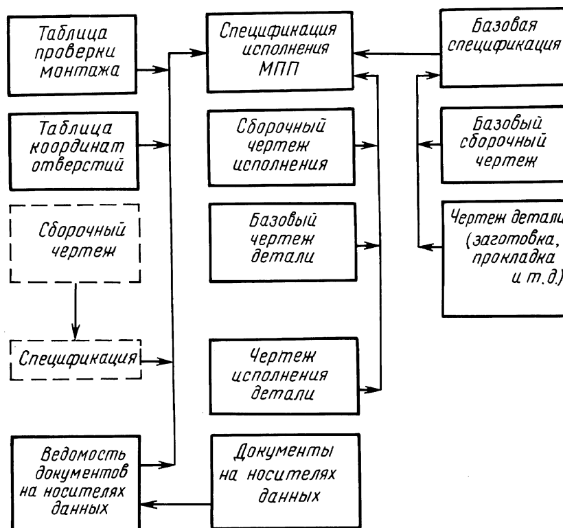
Пример построения комплекта конструкторских документов для МПП
