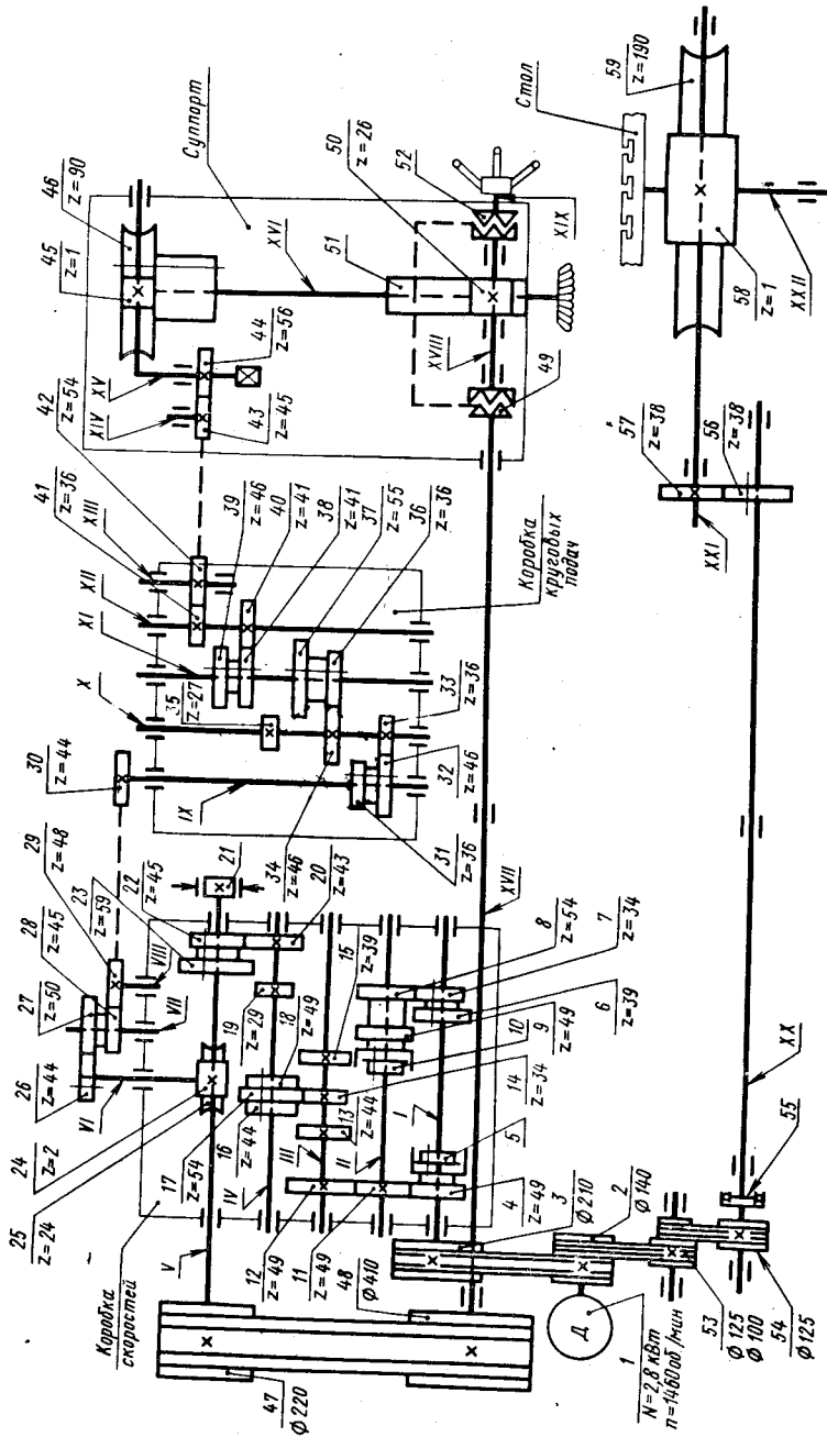
Пример выполнения кинематической схемы
